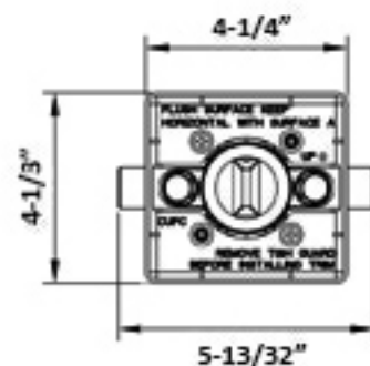
D1267200
