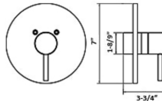
D2222201C / D2222201BN
