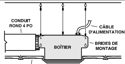
PLAFONDS SUSPENDUS Boîtier suspendu à des fils de fer en 3 points.
